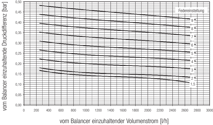
Einstellkurven Balancer G (DN 32)
